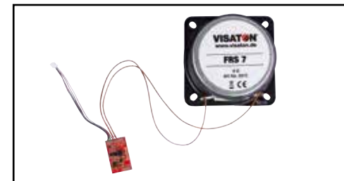
G-PSD XP 5.1 Sound mit Lautsprecher G-PSD XP 5.1 Sound with loud-speaker
