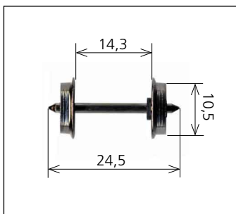
6048 Confezione 4 assali Ø 10,5 mm. Box of 4 axles Ø 10,5 mm.
