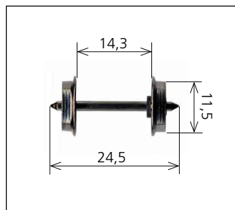
6047 Confezione 4 assali Ø 11,5 mm. Box of 4 axles Ø 11,5 mm.
