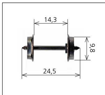
6049 Confezione 4 assali Ø 9,8 mm. Box of 4 axles Ø 9,8 mm.
